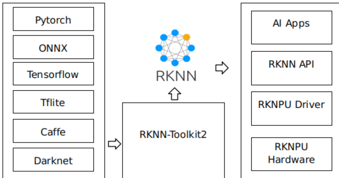
图 1-1 RKNN 软件栈
