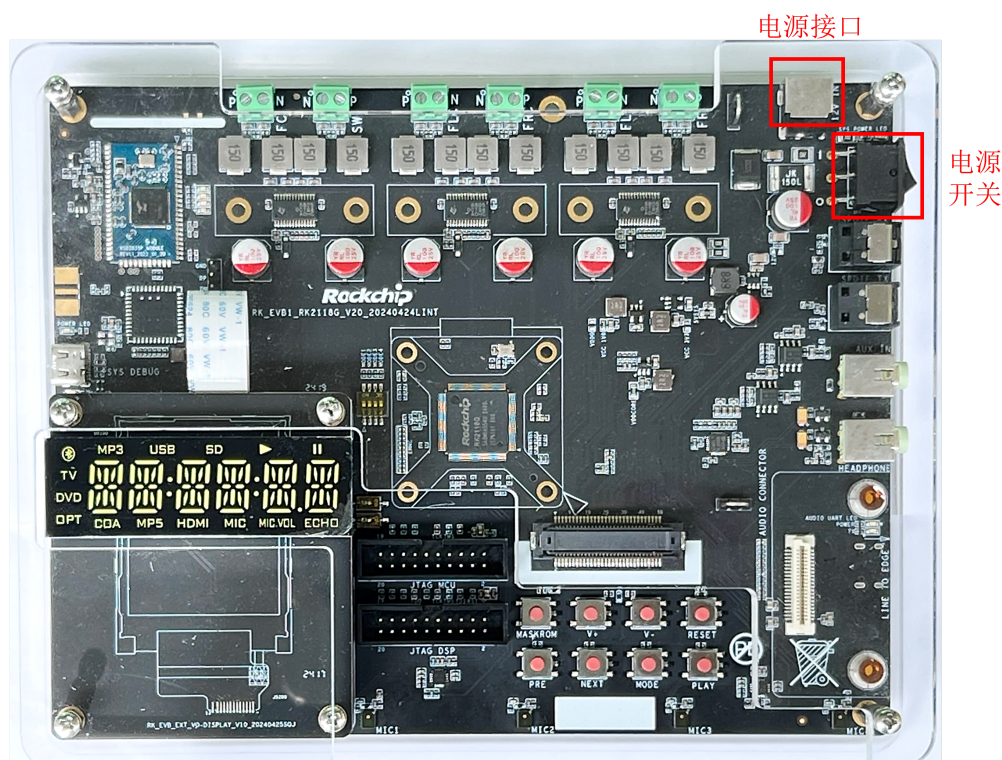
图2-1 RK2118开发板
