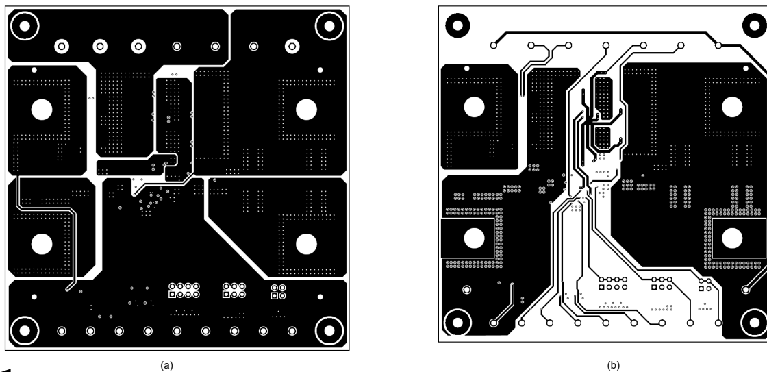
图 6-3. TPS48111Q1EVM 电路板 (a) 内部信号层 (b) 内部布线层
